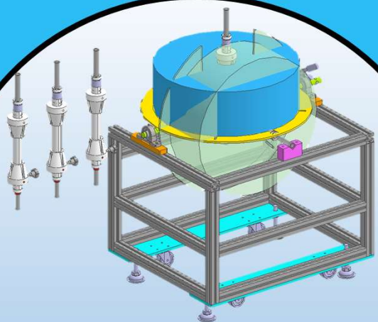
前段取り替え治具 シャフト3本
